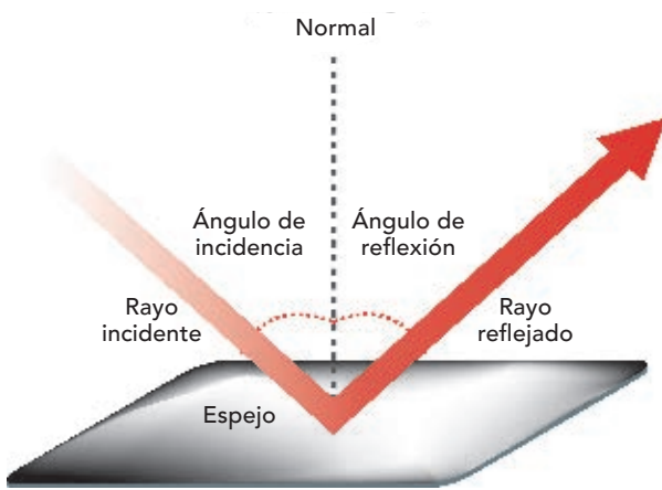
Reflexión de la luz.
