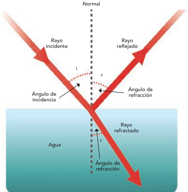
Refracción de la luz.
